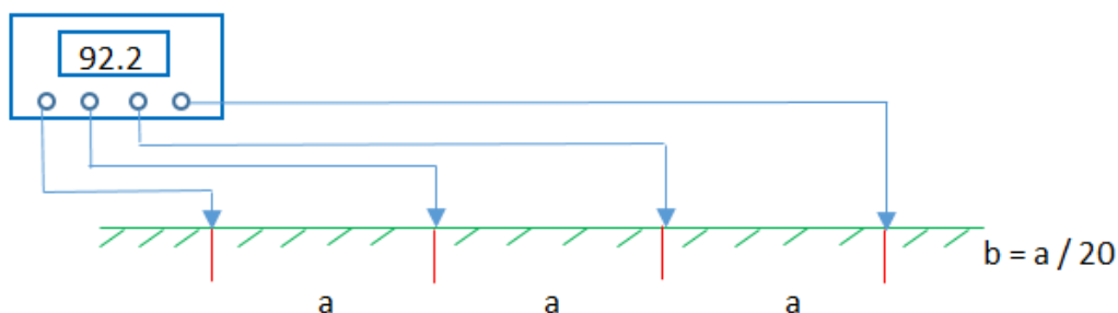
Figura 9. Diagrama de conexión del telurómetro METREL MI-3123 para efectuar la medida de resistividad del terreno en el municipios de Maicao, La Guajira, utilizando el método de los cuatro puntos de WENNER
