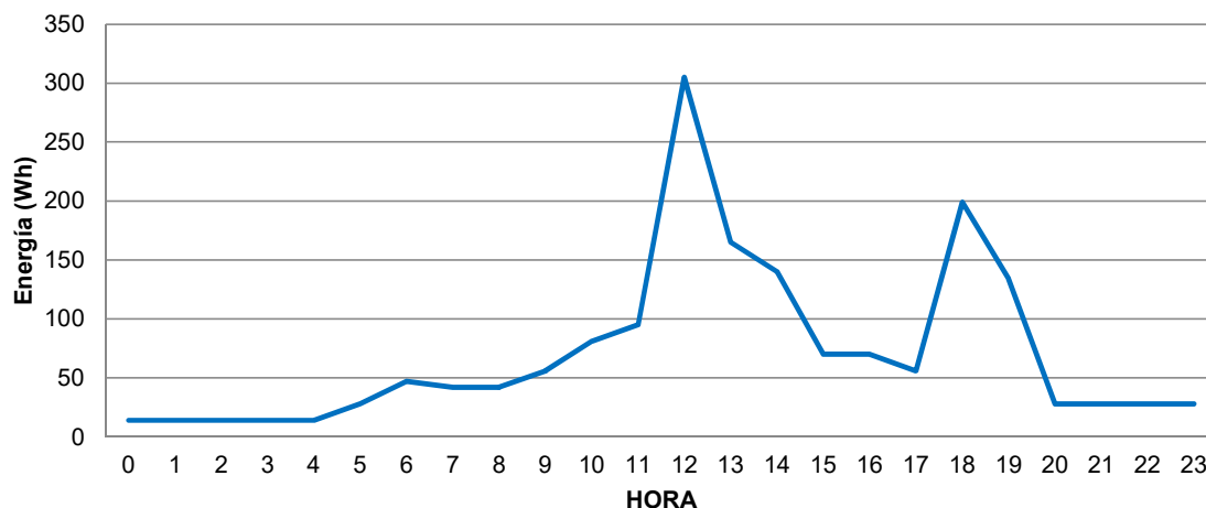
Figura 3. Curva de carga horaria diaria inicial de una UCA rural dispersa en el municipio de Maicao, La Guajira
