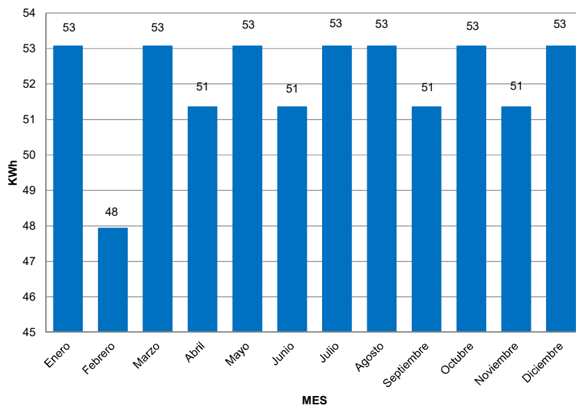
Figura 4. Gráfico del consumo mensual inicial para una UCA rural dispersa en el municipio de Maicao, La Guajira
