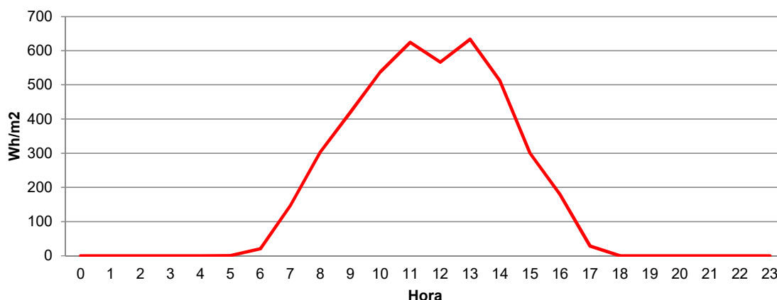
Figura 6. Curva de radiación solar promedio horaria diaria inclinada a 11^\circ en el mes de noviembre en el Municipio de Maicao, La Guajira del “Atlas de Radiación Solar, Ultravioleta y Ozono de Colombia”
