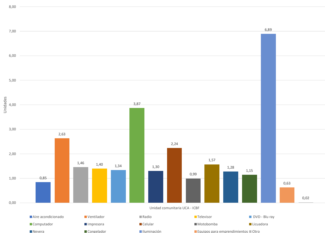
Figura 2. Necesidades energéticas promedio arrojadas por las encuestas para las UCAS rurales en las ZNI del municipio de Maicao, La Guajira
